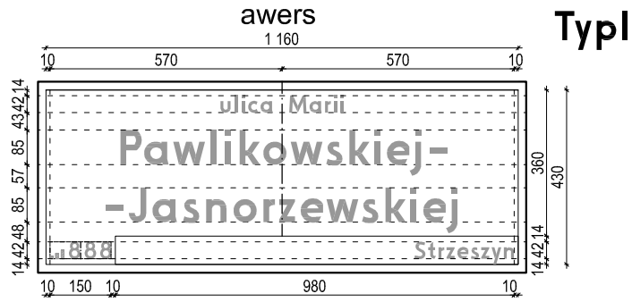
zał.6 rys.7a - Wymiary tablic mocowanych na elewacji - w prawym narożu budynku
