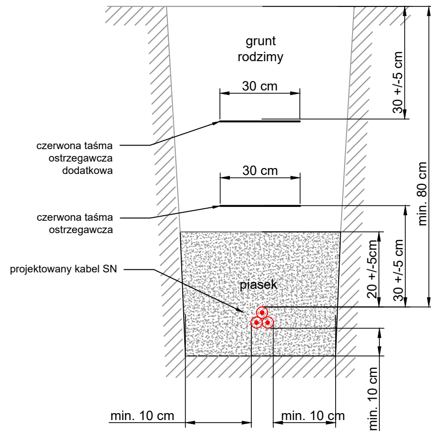
PRZEKRÓJ PROJEKTOWANEJ LINII KABLOWEJ SN-15kV W WYKOPIE
