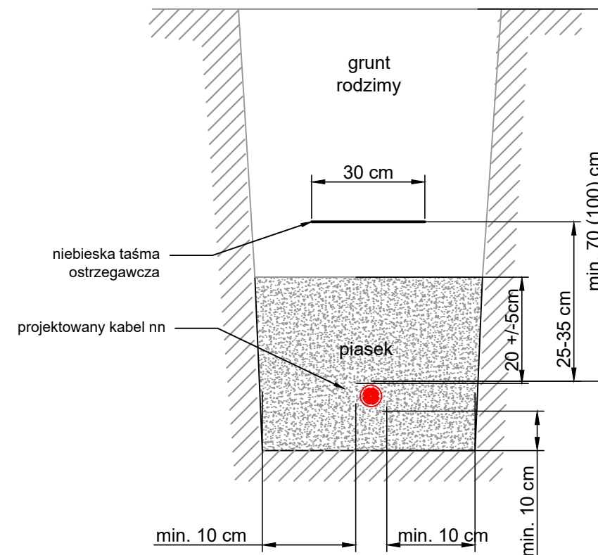
PRZEKRÓJ PROJEKTOWANEJ LINII KABLOWEJ nn-0,4kV W WYKOPIE
