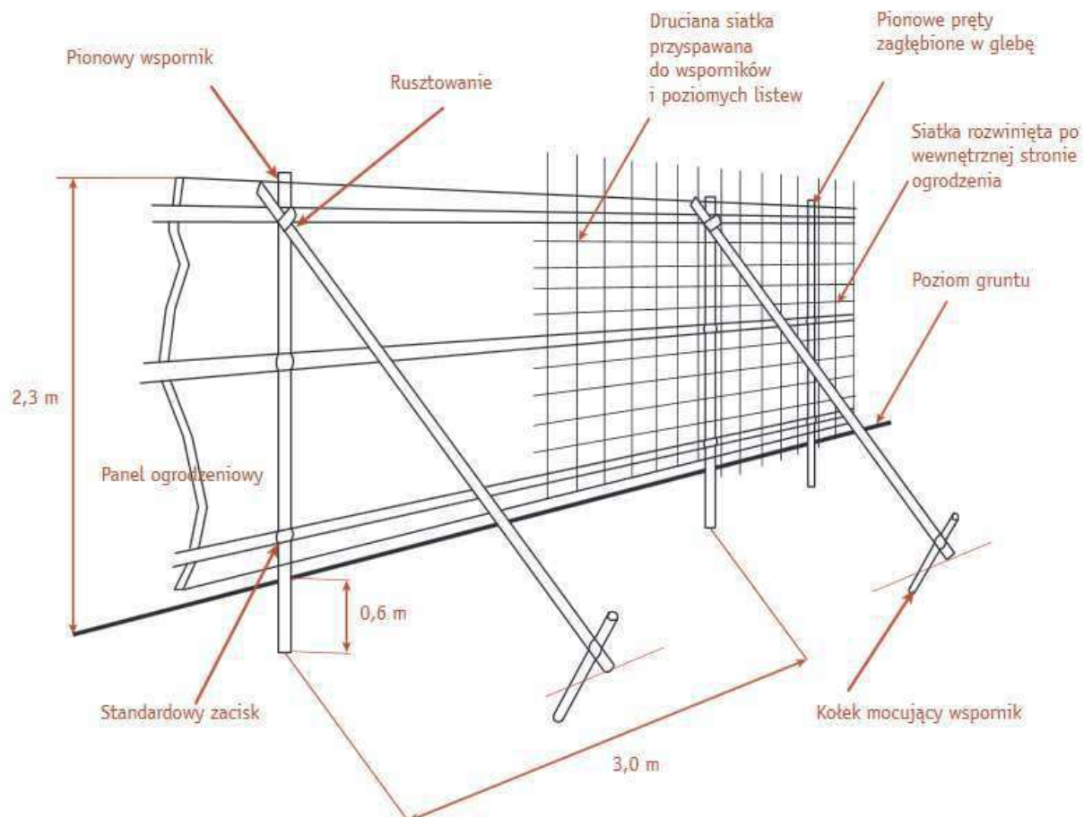
Ryc.1. Trwałe wygradzenia ochronne – przykładowa konstrukcja.
