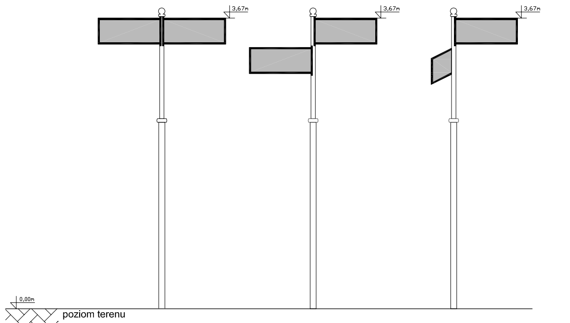
zał.2 rys. 5a - Schemat umieszczania tabliczek na konstrukcji wsporczej
