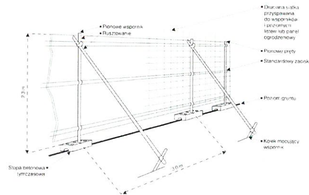
PRZYKŁAD OGRODZENIA OCHRONNEGO WEDŁUG BS 5837:2012. ZMODYFIKOWANY
