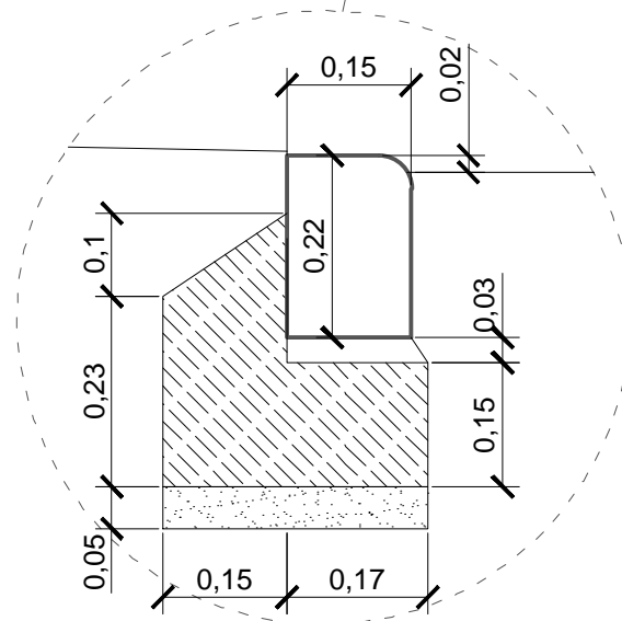
DETAL - KRAWĘŻNIK OBNIŻONY
