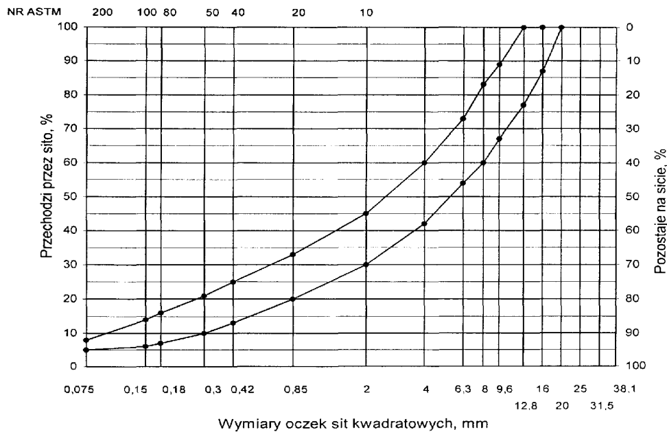
ys. 13. Krzywe graniczne uziarnienia mieszanki mineralnej BA od 0 do 16 mm do warstwy wyrównawczej nawierzchni drogi o obciążeniu ruchem od KR3 do KR6
